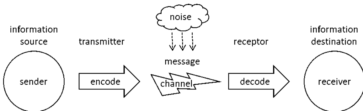
Abbildung 25: Das Shannon-Weaver-Kommunikationsmodell
